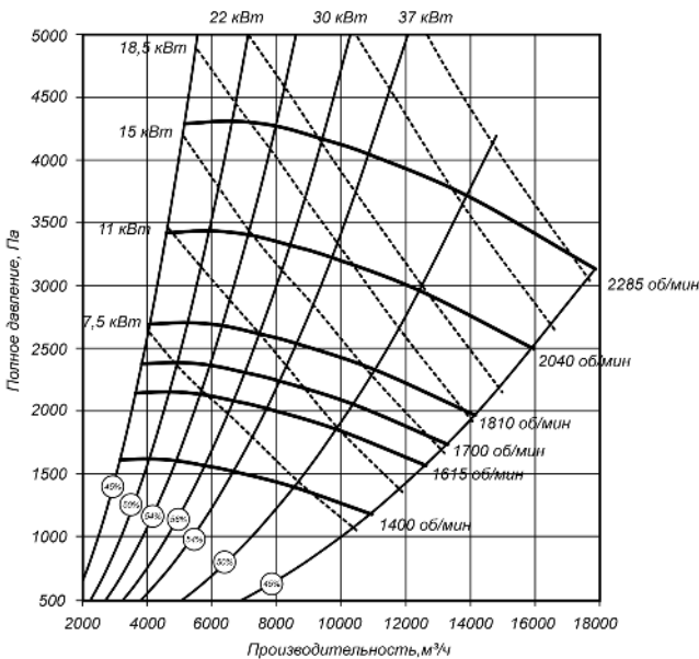
Аэродинамические характеристики ВЦП 7-40-6,3, исполнение 5
