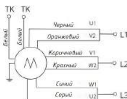
По схеме "треугольник"
