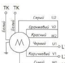
По схеме "звезда"
